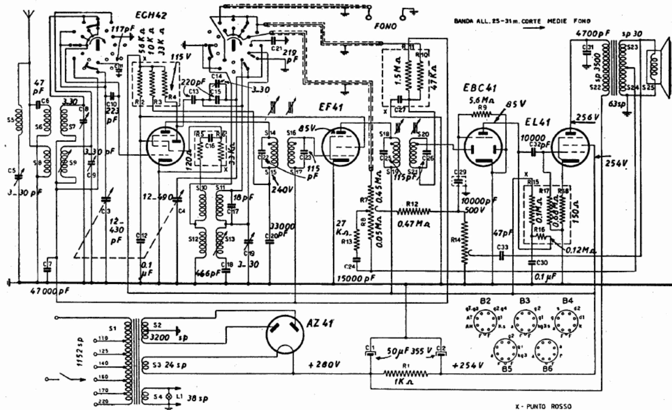
PHILIPS RADIO - Mod. BI. 310 A - Media frequenza 468 kc. Taratura OC a 16,5 Mc, ed a 6 Mc; banda allargata a 9,4 Mc. Onde medie a 1650 kc ed a 550 kc.
